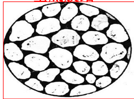
孔隙胶结
