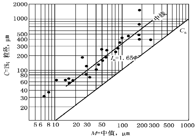
浊流沉积C—M图
