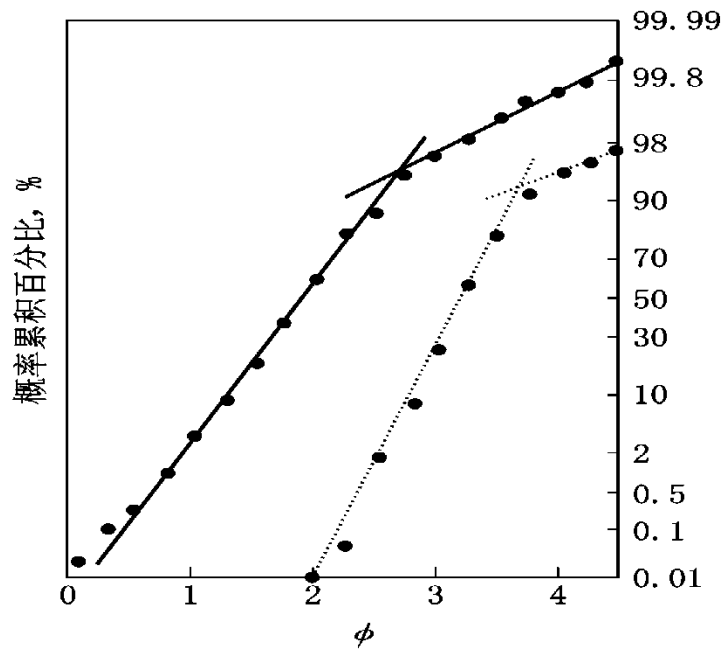
现代河道砂的粒度概率图
