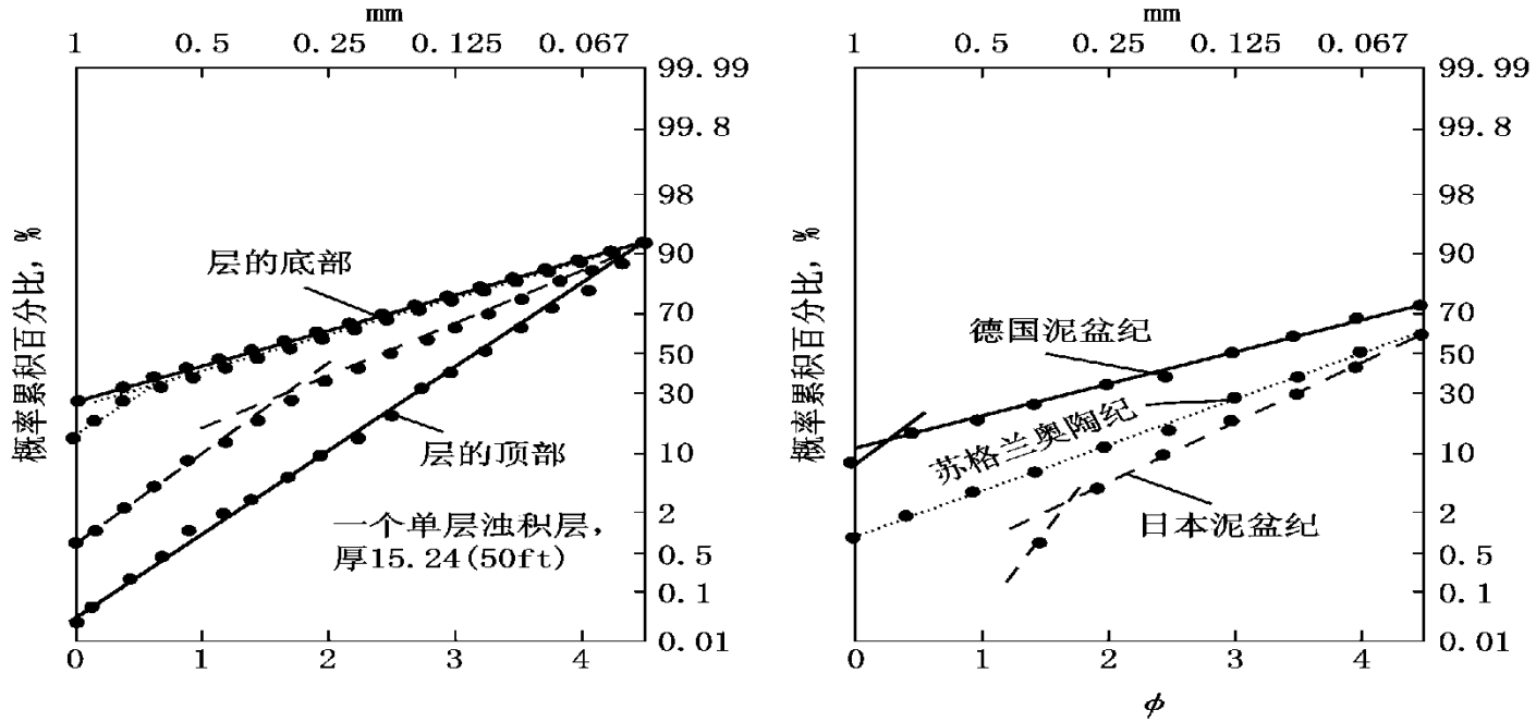
浊流沉积的粒度概率图
