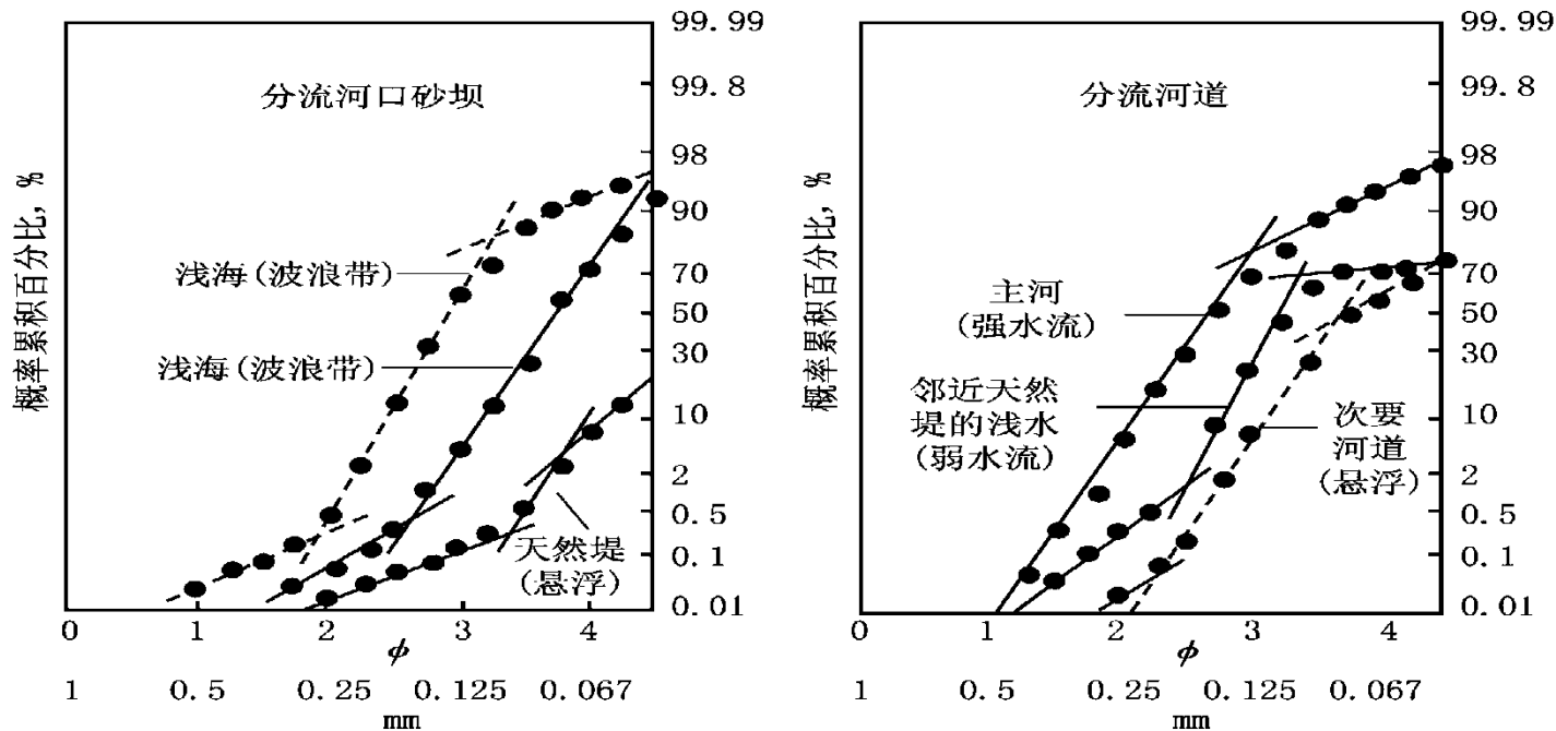
支流河口沙坝及支流河道砂的粒度概率图
