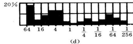
图 4-9 不同成因碎屑沉积物的粒度组分直方图 (转引自 H.B. 瓦索也维奇, 1958)
