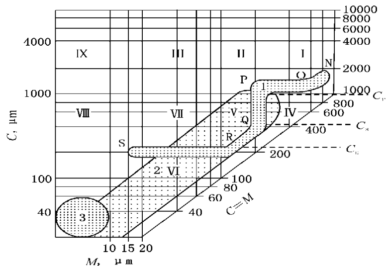
1.牵引流沉积；2.油流沉积；3.静水悬浮沉积
