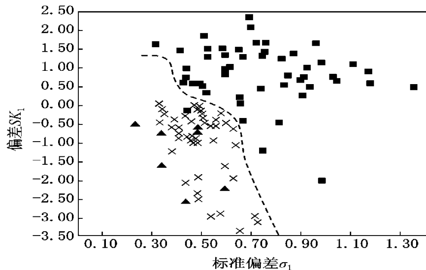
偏度与标准偏差结构参数散点图
