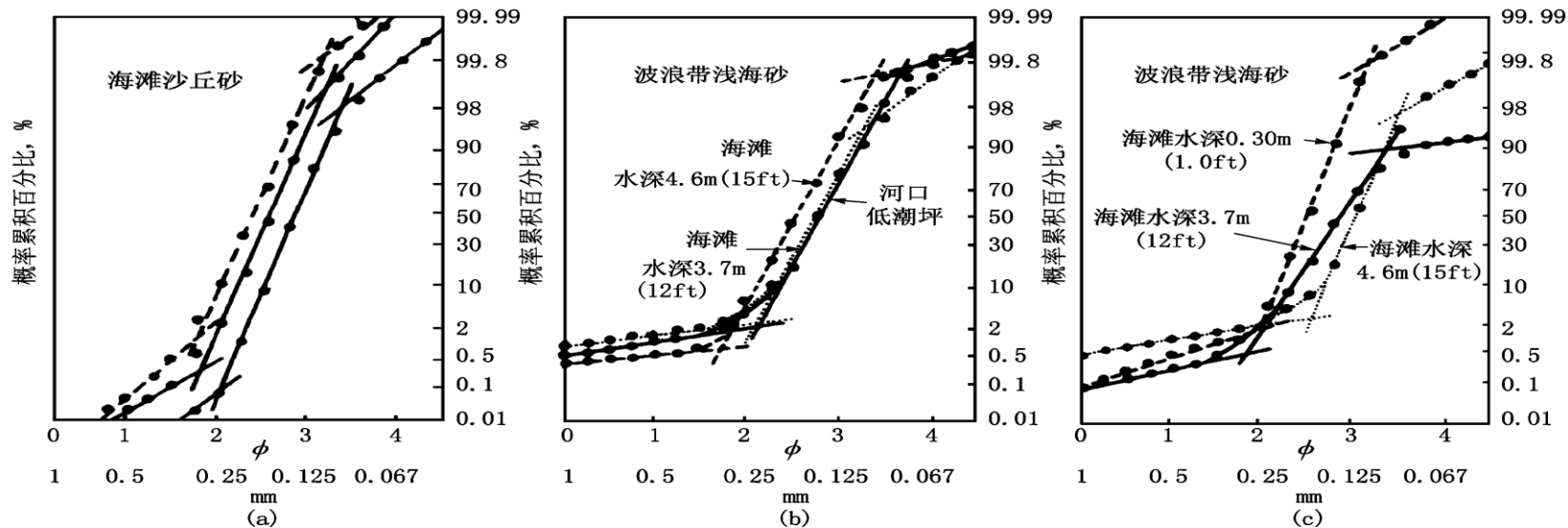
海滩砂丘砂和波浪带浅海砂的粒度概率图
