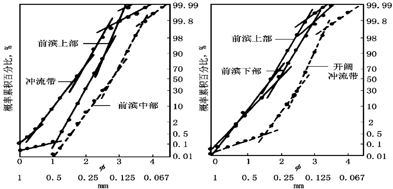
海滩砂的粒度概率图
