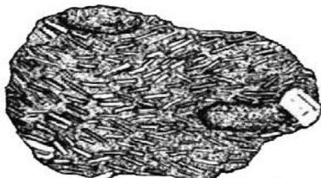
碱性喷出岩
