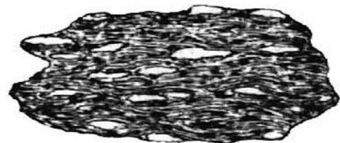
千枚岩
