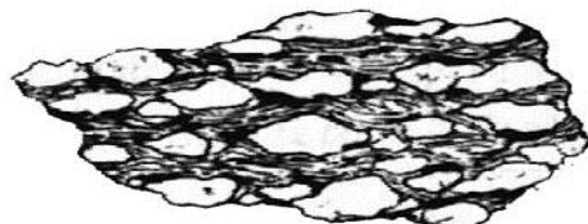
片岩
