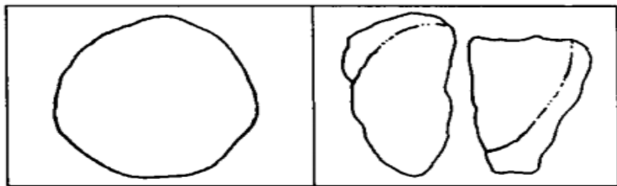
图 3-3 再旋回石英
