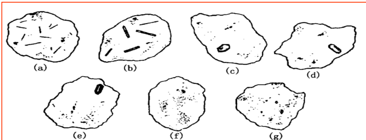
图 3-1 岩浆岩中的石英包裹体
