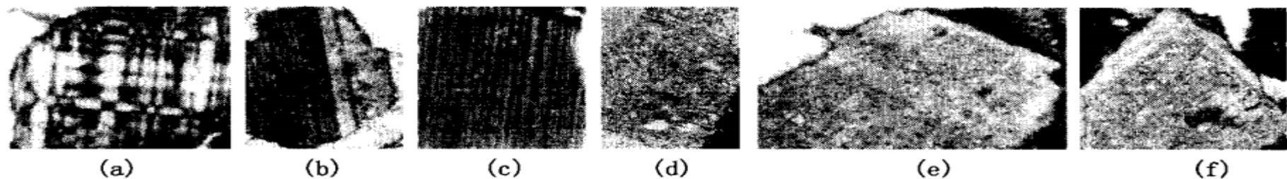
图 3-4 各种碎屑长石
