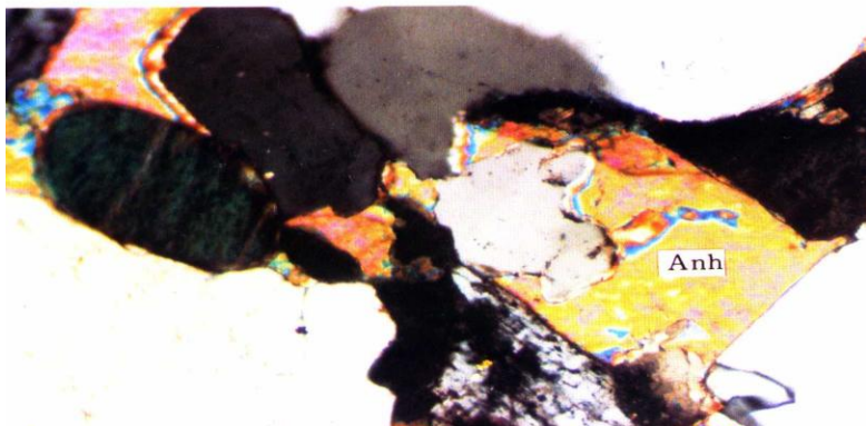
硬石膏胶结物
