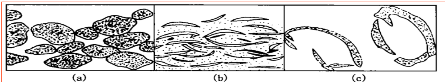
图 3-6 盆内碎屑 (刘孟慧素描)
