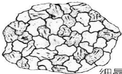
细晶岩
