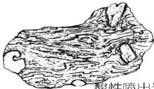
酸性喷出岩
