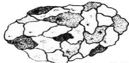
变质石英岩
